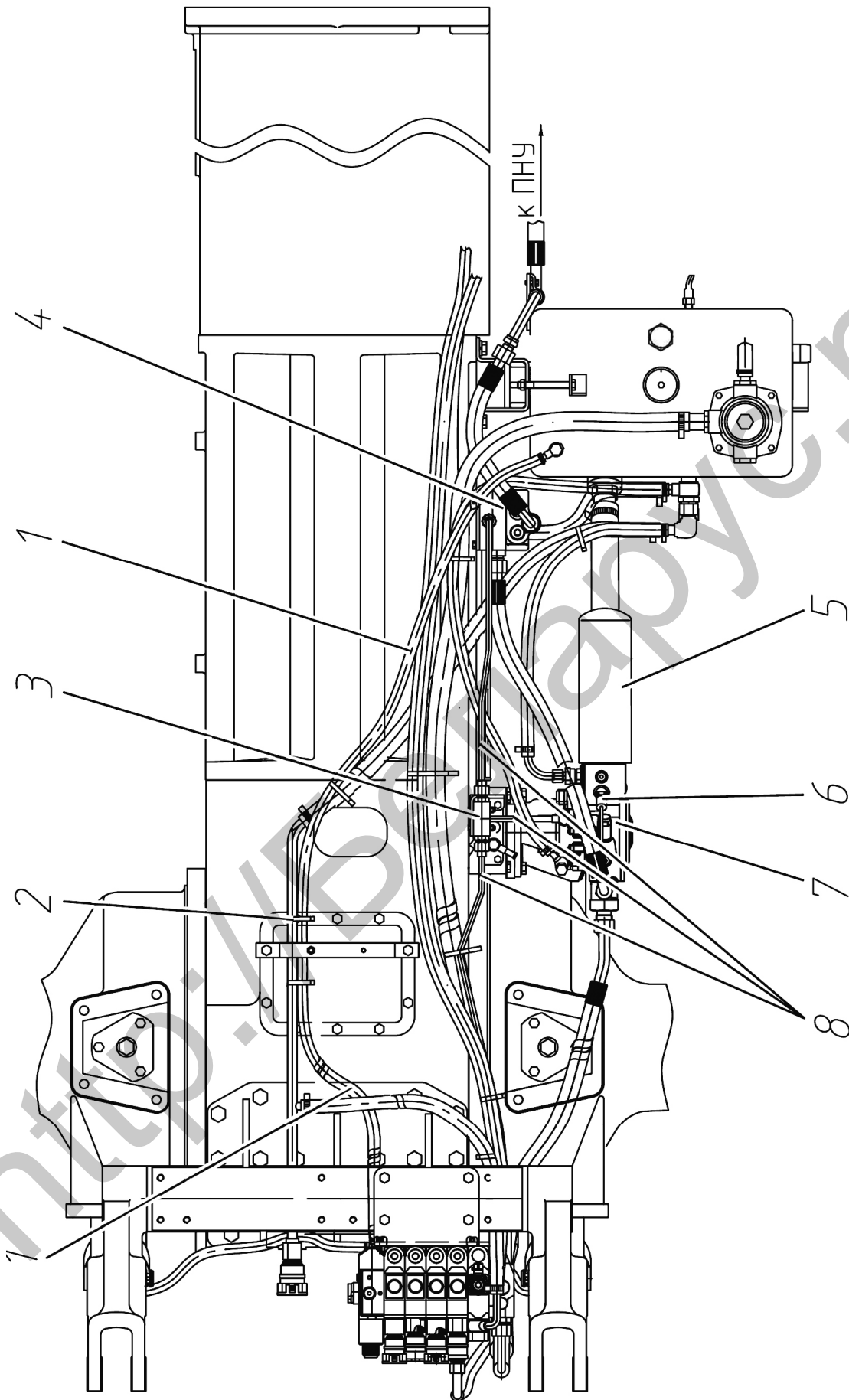
1 – магистраль дренажная гидроцилиндров; 2 – магистраль свободного слива (заднего); 3 – клапан "ИЛИ"; 4 – электро-гидравлический регулятор управления ПНУ; 5 – сменный фильтр регулируемого насоса; 6 – датчик засоренности; 7 – насос регулируемый; 8 – магистраль канала управления.
