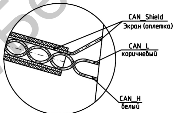
Рисунок 7.14.2 – Структура CAN кабеля
