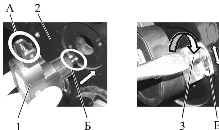
1 – позиционный датчик; 2 – кронштейн ПНУ; 3 – винт. Рисунок 3.16.13 – Установка позиционного датчика ПНУ
