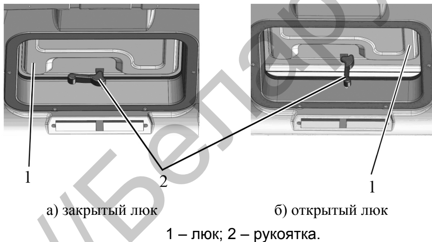
Рисунок 2.18.5 – Открытие люка с рукояткой
