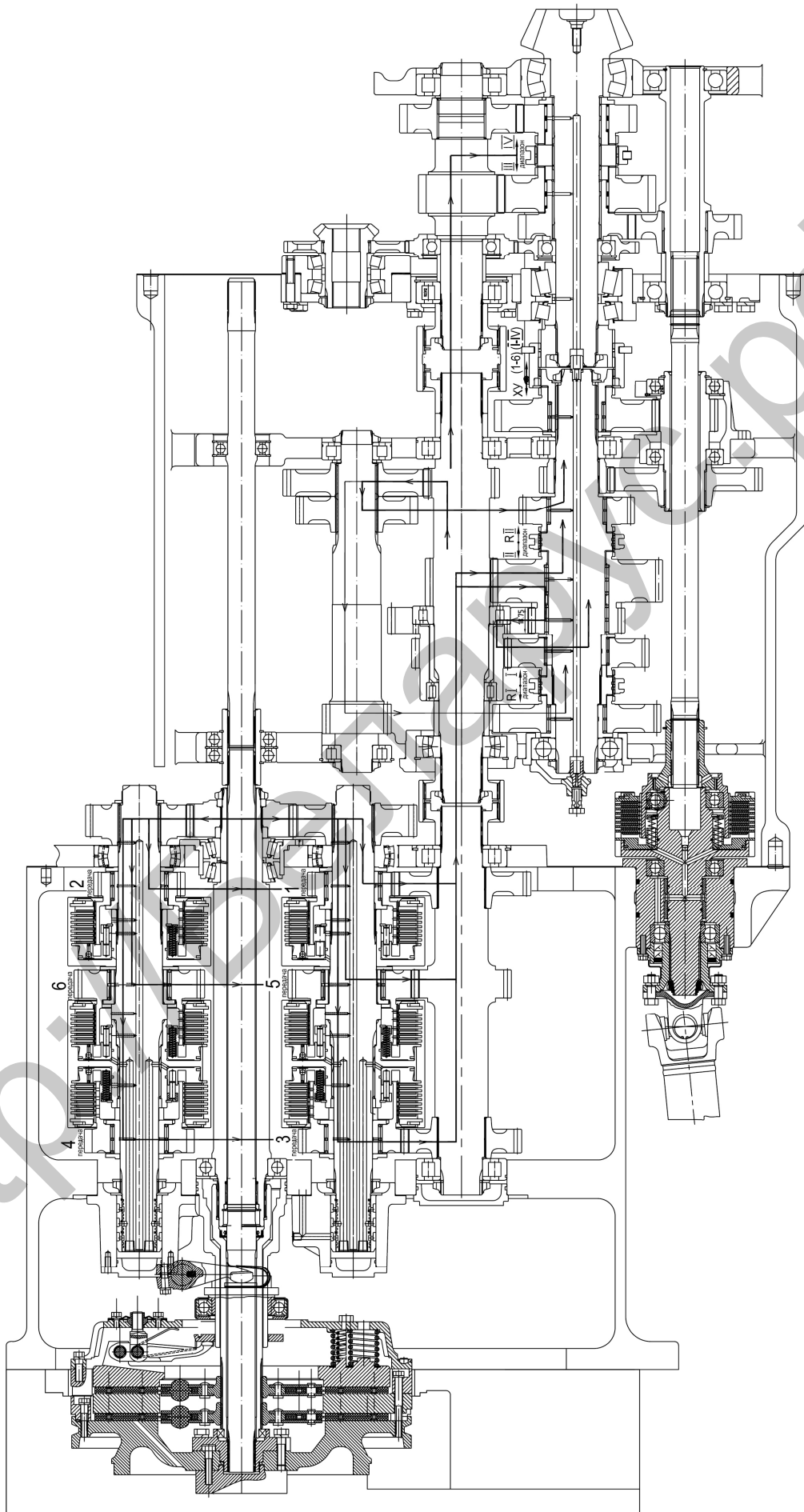
Рисунок 3.4.6 — Схема направлений силовых потоков передач по диапазонам
