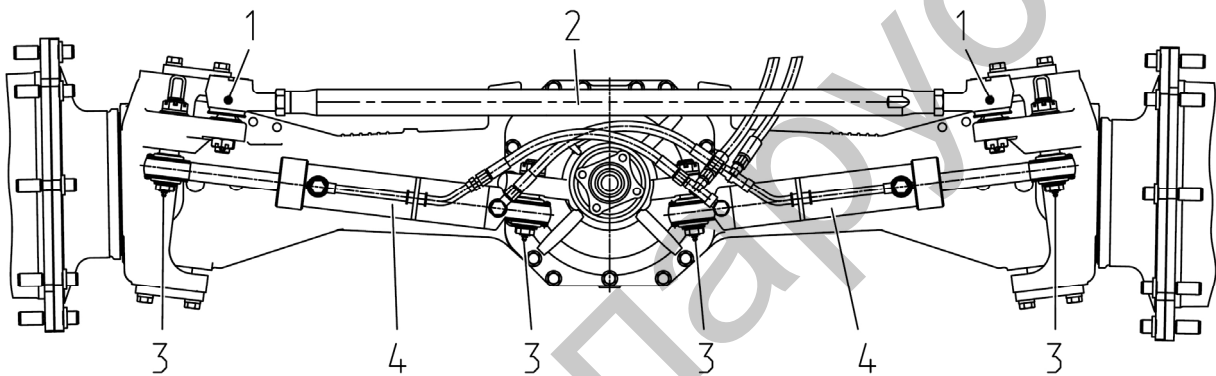
1, 3 – масленка; 2 – рулевая тяга; 4 – гидроцилиндр ГОРУ.
