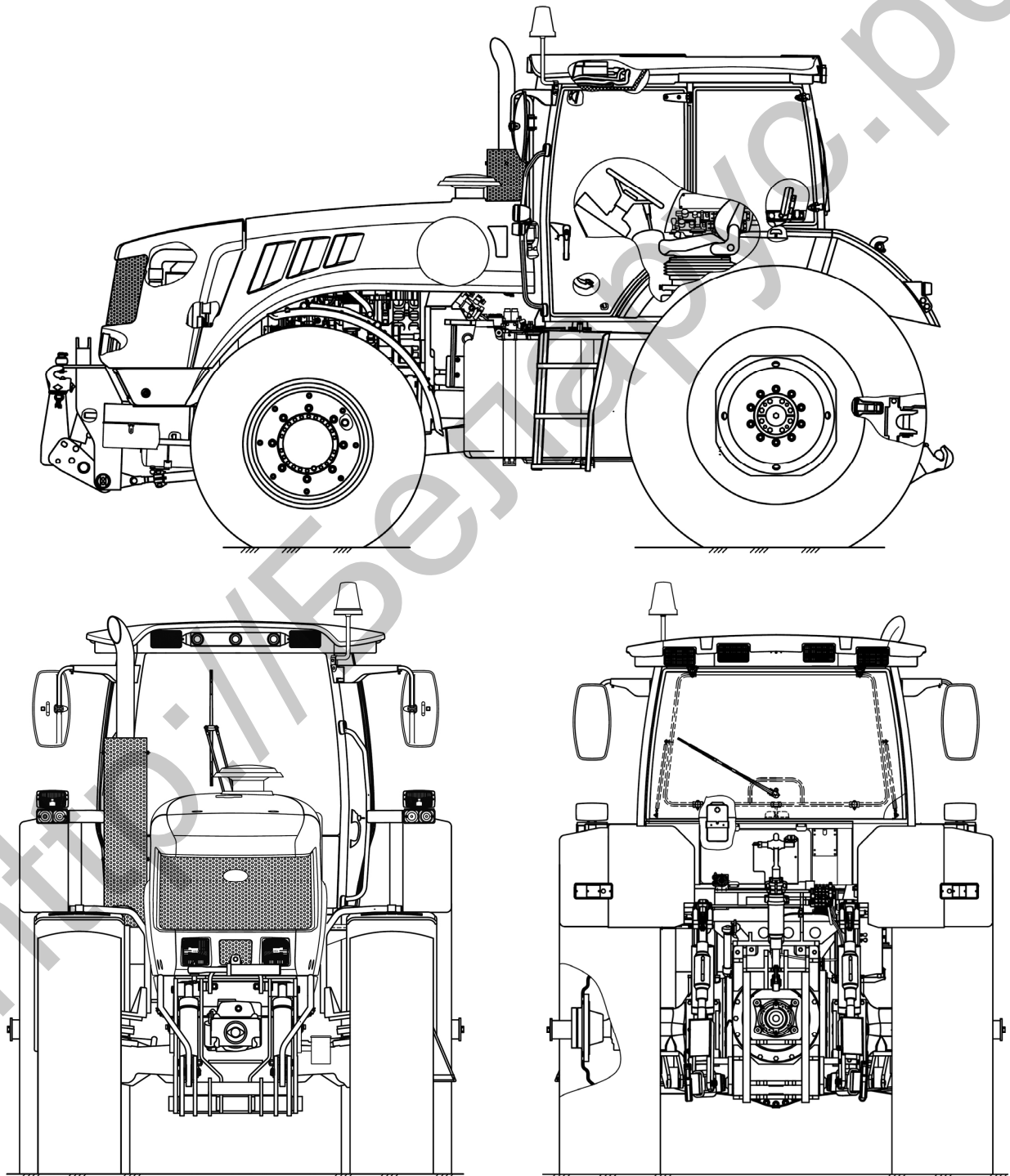
Рисунок 1.1.1 – Трактор «БЕЛАРУС-3022ДЦ.1»
