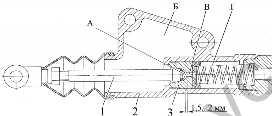
Рисунок 3.9.6 – Главный тормозной цилиндр реверса
