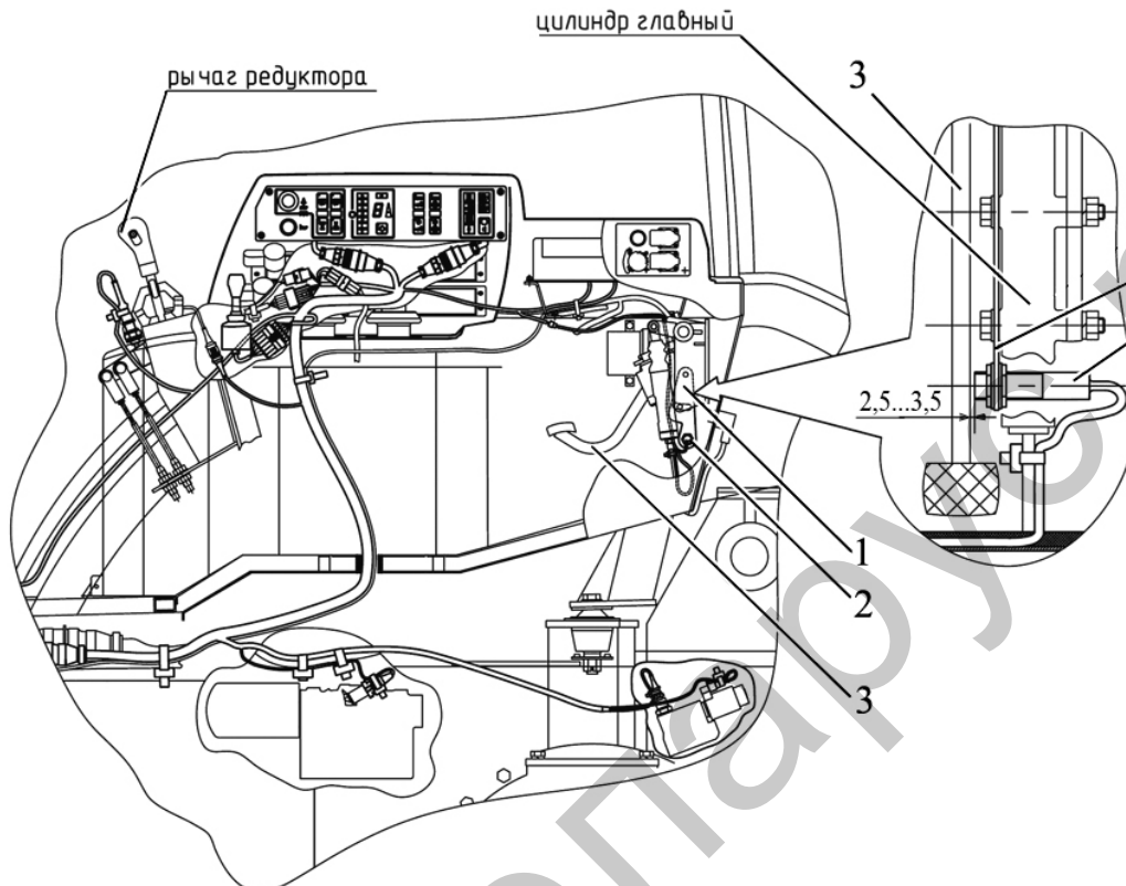
Рисунок 3.5.3 – Установка датчика выключенного состояния сцепления на реверсе
