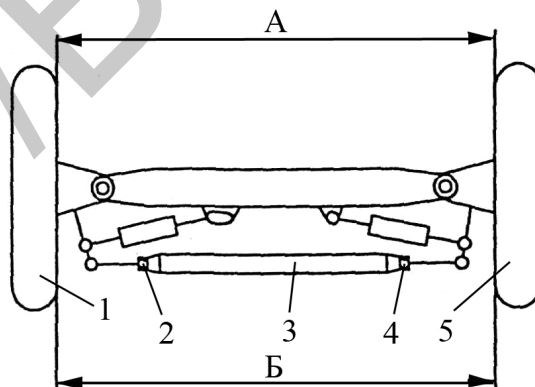
Рисунок 6.4.34 – Схема регулировки сходимости передних колес
