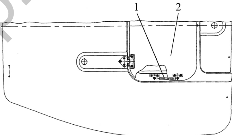
1 – пневмоподъемник; 2 – люк.
