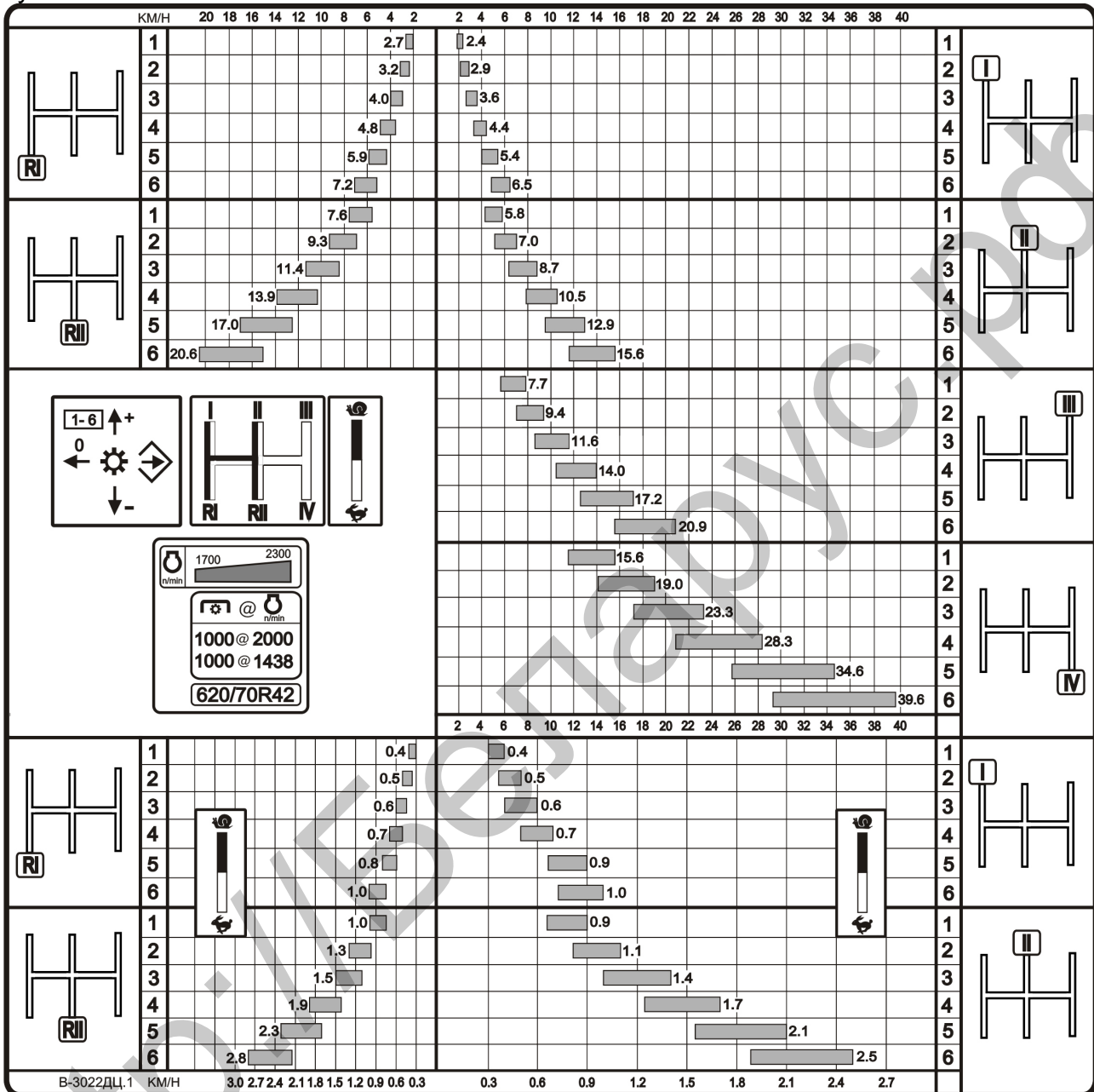
Рисунок 2.13.3 – Диаграмма скоростей трактора «БЕЛАРУС-3022ДЦ.1»
