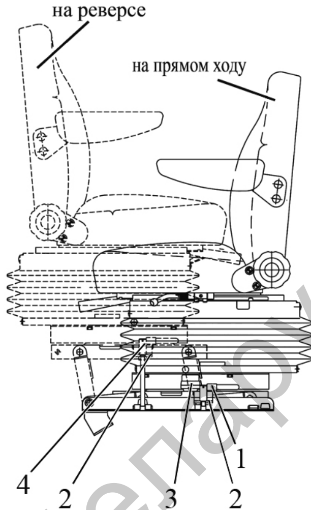
Рисунок 2.19.2 – Установка сиденья для работы на реверсивном ходу
