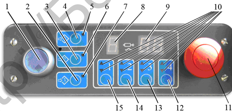
Рисунок 4.2.3 – Управление секциями гидрораспределителя EHS
