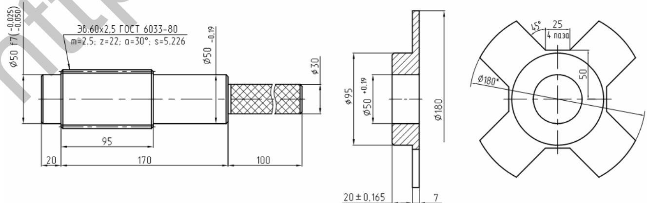
Рисунок 3.3.3 – Технологическая оправка
