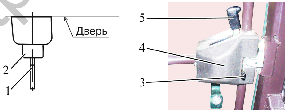
1 – ключ замка; 2 – кнопка замка; 3, 5 – рукоятка; 4 – замок.
