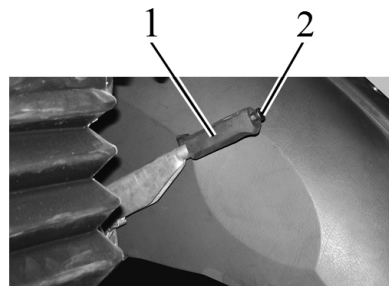
Рисунок 2.11.1 – Управление стояночным тормозом
