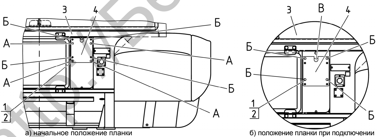
Рисунок 2.20.2 – Установка электрических розеток и прикуривателя
