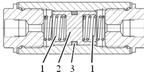
Рисунок 3.9.4 – Уравнительный клапан
