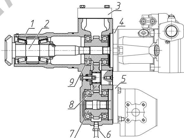
Рисунок 3.16.7 – Привод насосов
