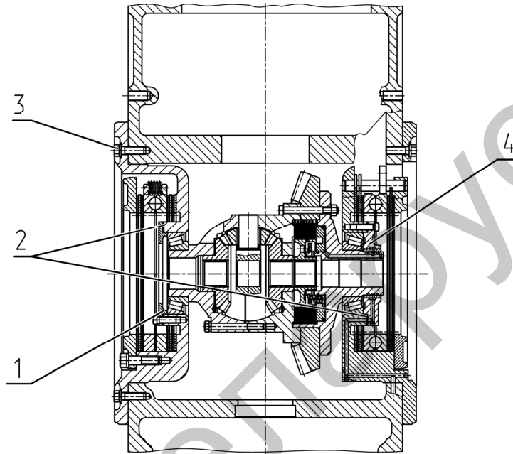
Рисунок 3.6.4 – Дифференциал в корпусе заднего моста
