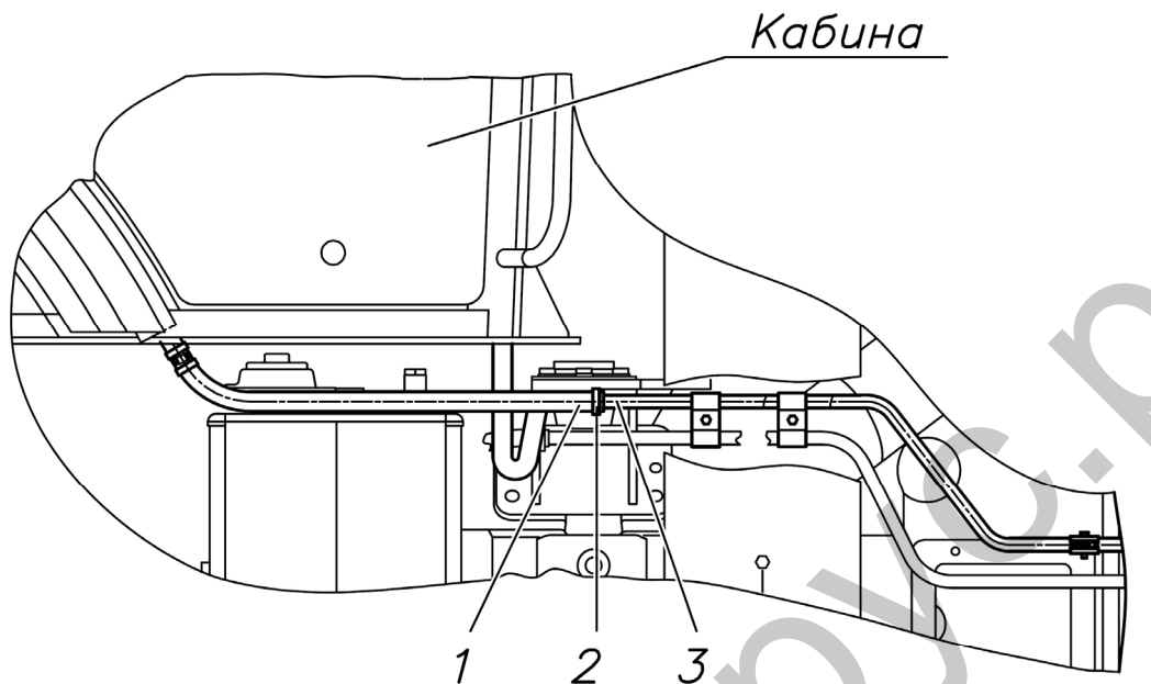
а) Вид справа
